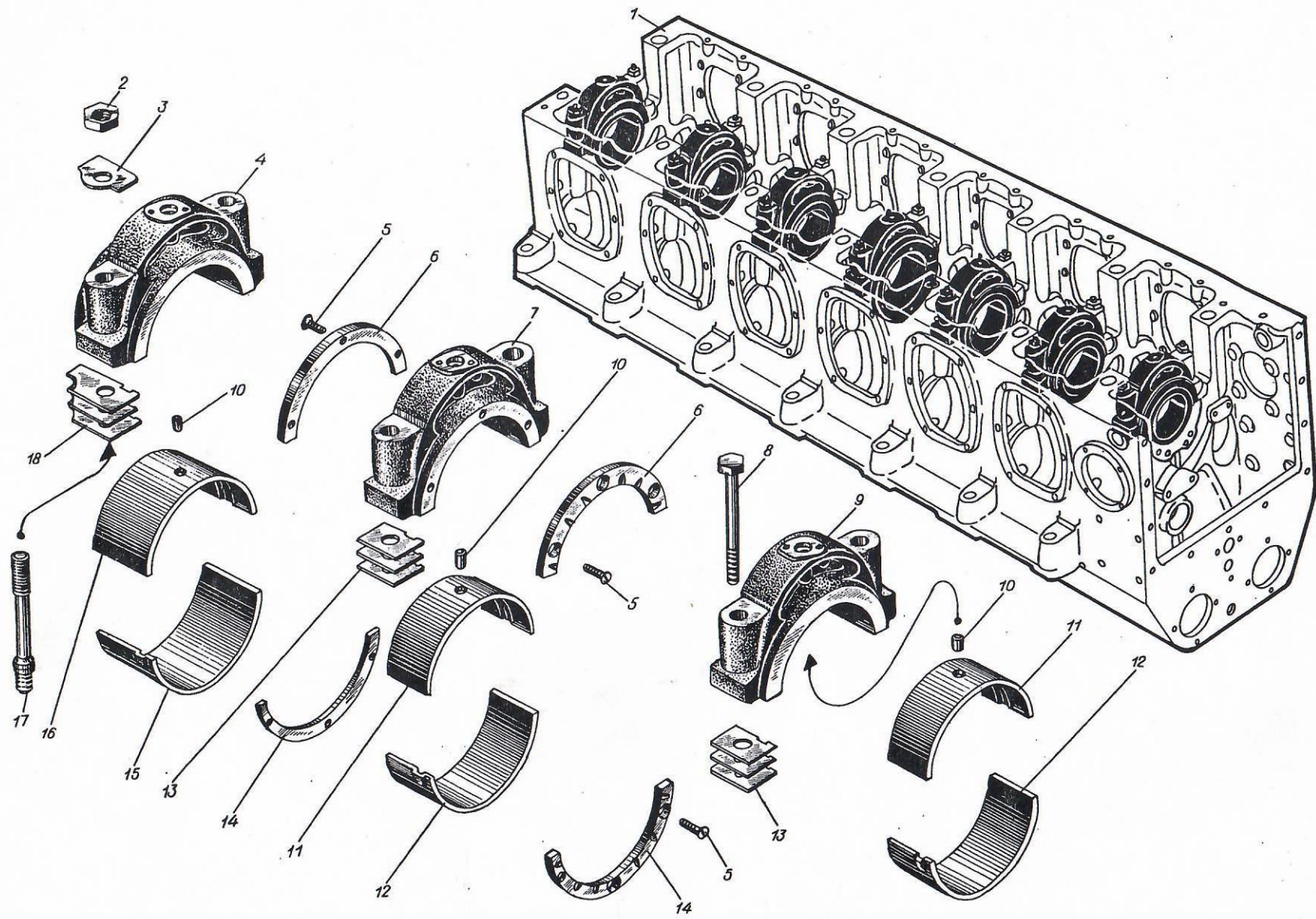
Рис. 2. Рама фундаментная. Подшипники коленчатого вала Fig. 2. Foundation frame. Crankshaft bearings
